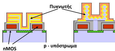
Πυκνωτές Επιφανείας
