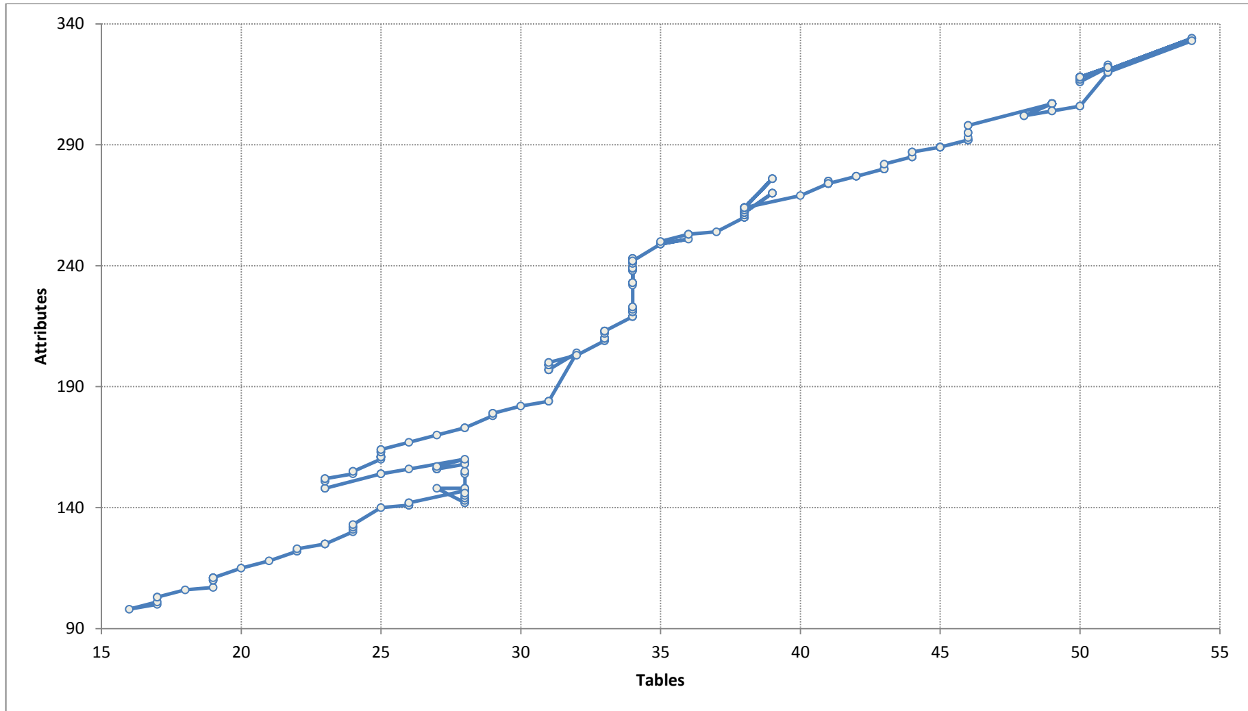
b) Timeline for MediaWiki
