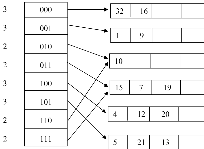
Εικόνα 10.6 Επεκτατός Δυναμικό Κατακερματισμός
