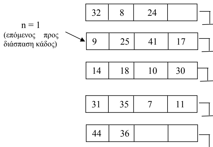
Εικόνα 10.15 Γραμμικός Κατακερματισμός, έχει διασπαστεί ο κάδος 0
