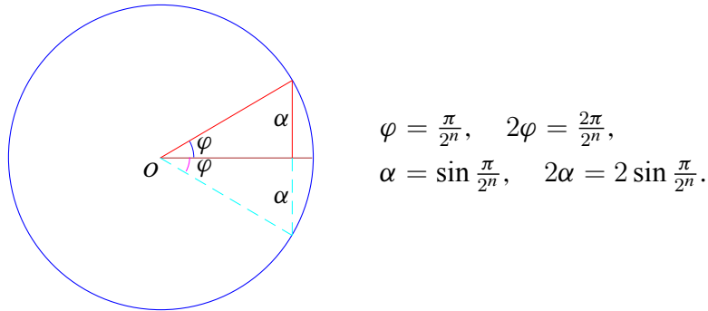
Figure 1: Το εγγεγραμμένο στον μοναδιαίο κύκλο κανονικό πολύγωνο με 2^n πλευρές έχει πλευρά 2\alpha = 2 \sin \frac{\pi}{2^n} και περίμετρο 2^n \cdot 2 \sin \frac{\pi}{2^n} = 2y_n .
