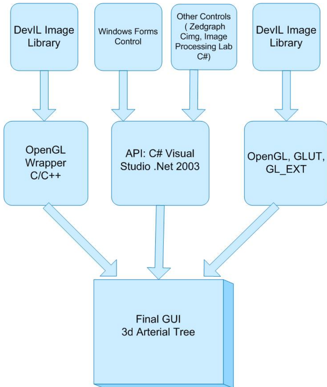
Σχήμα 4.1 Διάγραμμα Ανάπτυξης Λογισμικού
