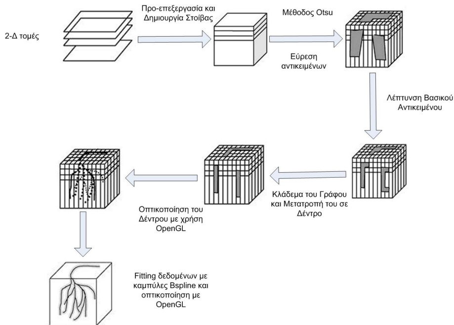
Σχήμα 3.1. Βήματα Μεθοδολογίας που Ακολουθείται
