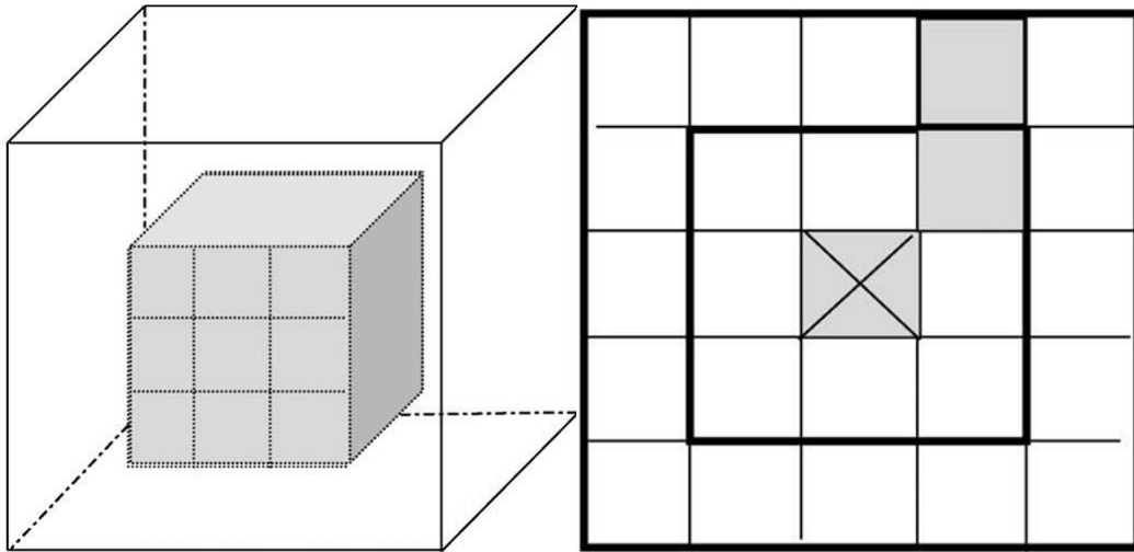
Σχήμα 3.19 Παράδειγμα line end voxel
