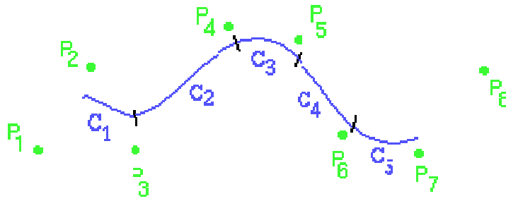
Σχήμα 3.21 Μια καμπύλη B-spline τρίτου βαθμού με 8 σημεία ελέγχου
