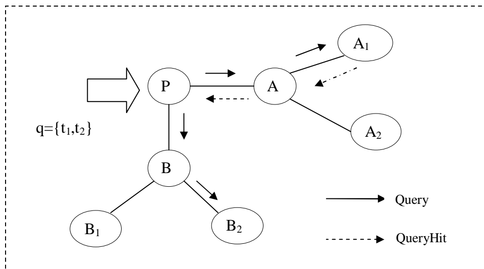
Σχήμα 2.1 Παράδειγμα εκτέλεσης του Forward μηχανισμού αναζήτησης. Ο P υποβάλει την ερώτηση q à ία χρονική στιγμή t . Ο A_1 είναι ο à οναδικός κόμβος στο δίκτυο που έχει στη LDC του έγγραφα που ικανοποιούν την q
