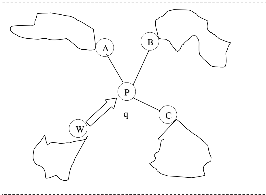
Σχήμα 2.2 Το πρόβλημα της επιλογής γειτόνων στο Forward σχήμα. Η πρώτη τυχαία επιλογή του P για μια q θα επηρεάσει \hat{} ελλοντικές q ' παρόμοιες της q με αποτέλεσμα κάποιες διαδρομές να μην εξερευνώνται ποτέ
