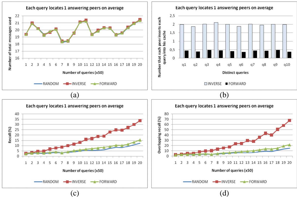
Σχήμα 3.3 Σε δίκτυο με 1000 κόμβους υποβάλλονται 10 ξεχωριστές ερωτήσεις που επαναλαμβάνονται 100 φορές η κάθε μια. Κάθε μια ξεχωριστή ερώτηση την πρώτη φορά που υποβάλλεται βρίσκει κατά μέσο όρο 1 κόμβο απάντησης. Οι παράμετροι του πειράματος απεικονίζονται στη στήλη 3.3.2 του πίνακα 3.2
