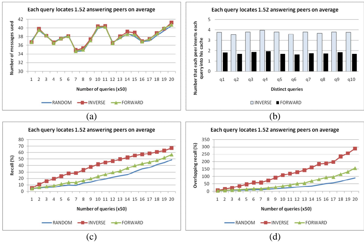
Σχήμα 3.4 Σε δίκτυο με 1000 κόμβους υποβάλλονται 10 ξεχωριστές ερωτήσεις που επαναλαμβάνονται 100 φορές η κάθε μια. κάθε μια ξεχωριστή ερώτηση την πρώτη φορά που υποβάλλεται βρίσκει κατά μέσο όρο 1.52 κόμβους απάντησης. Οι παράμετροι του πειράματος απεικονίζονται στη στήλη 3.3.3 του πίνακα 3.2
