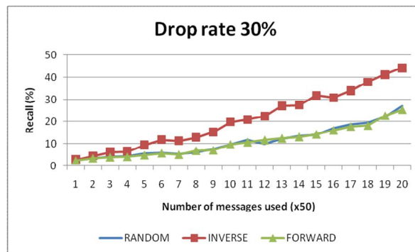
Σχήμα 3.6 Το recall για τα τρία σχήματα αναζήτησης στη \lambda έγιστη τιμή του drop rate ίση με 30%
