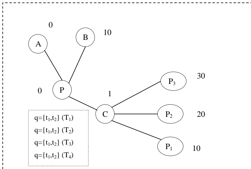
Σχήμα 2.3 Ο κόμβος C λαμβάνει σε 4 διαφορετικές χρονικές στιγμές T_1 , T_2 , T_3 και T_4 την ίδια ερώτηση q=\{t_1, t_2\} . Δίπλα σε κάθε κόμβο του δικτύου απεικονίζεται το πλήθος των εγγράφων που είναι σχετικά ως προς την q . Π.χ ο κόμβος A δεν έχει κανένα σχετικό έγγραφο ενώ ο κόμβος P_3 έχει 30
