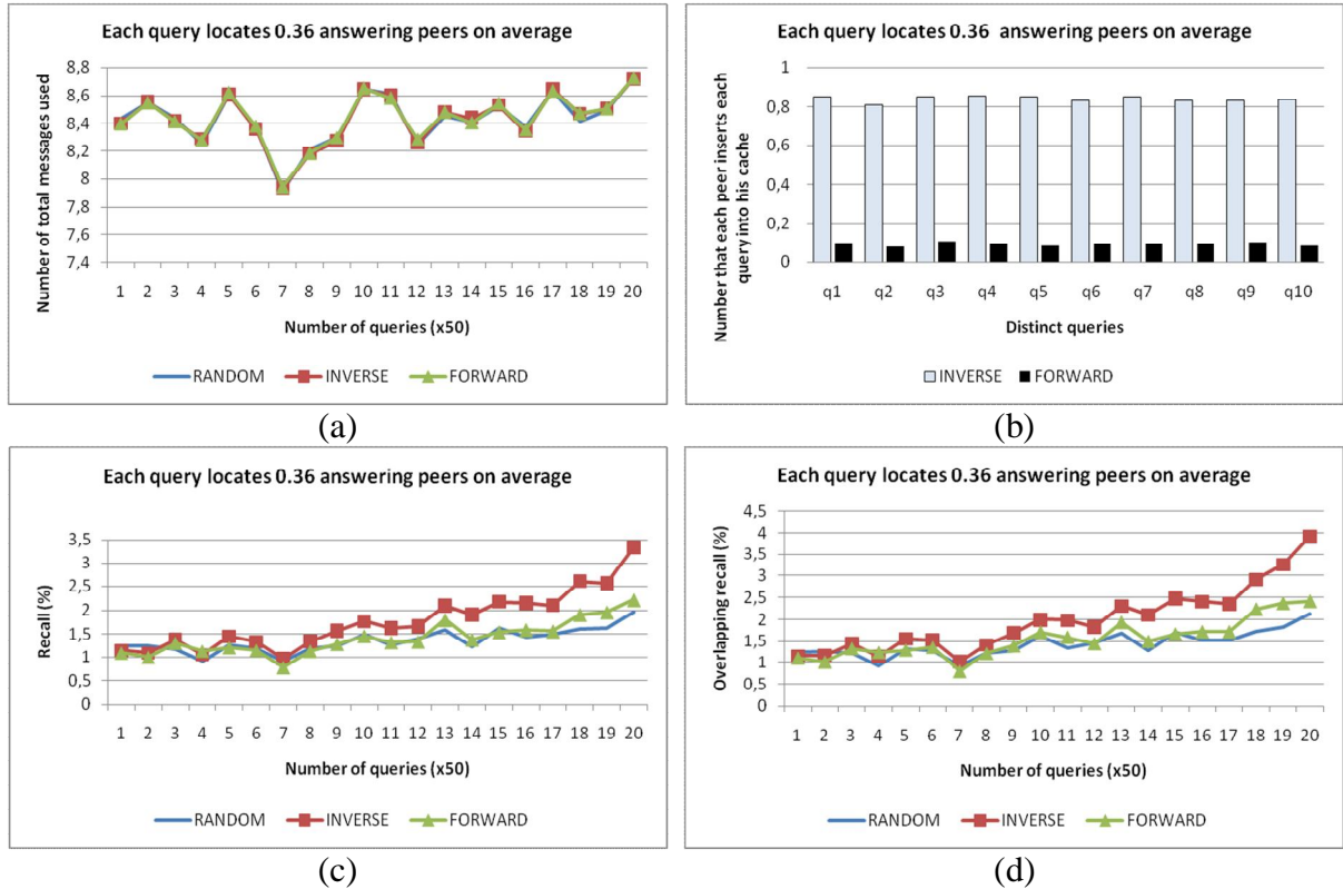
Σχήμα 3.2 Σε δίκτυο με 1000 κόμβους υποβάλλονται 10 ξεχωριστές ερωτήσεις που επαναλαμβάνονται 100 φορές η κάθε μια. Κάθε μια ξεχωριστή ερώτηση την πρώτη φορά που υποβάλλεται βρίσκει κατά μέσο όρο 0.36 κόμβους απάντησης. Οι παράμετροι του πειράματος απεικονίζονται στη στήλη 3.3.1 του πίνακα 3.2
