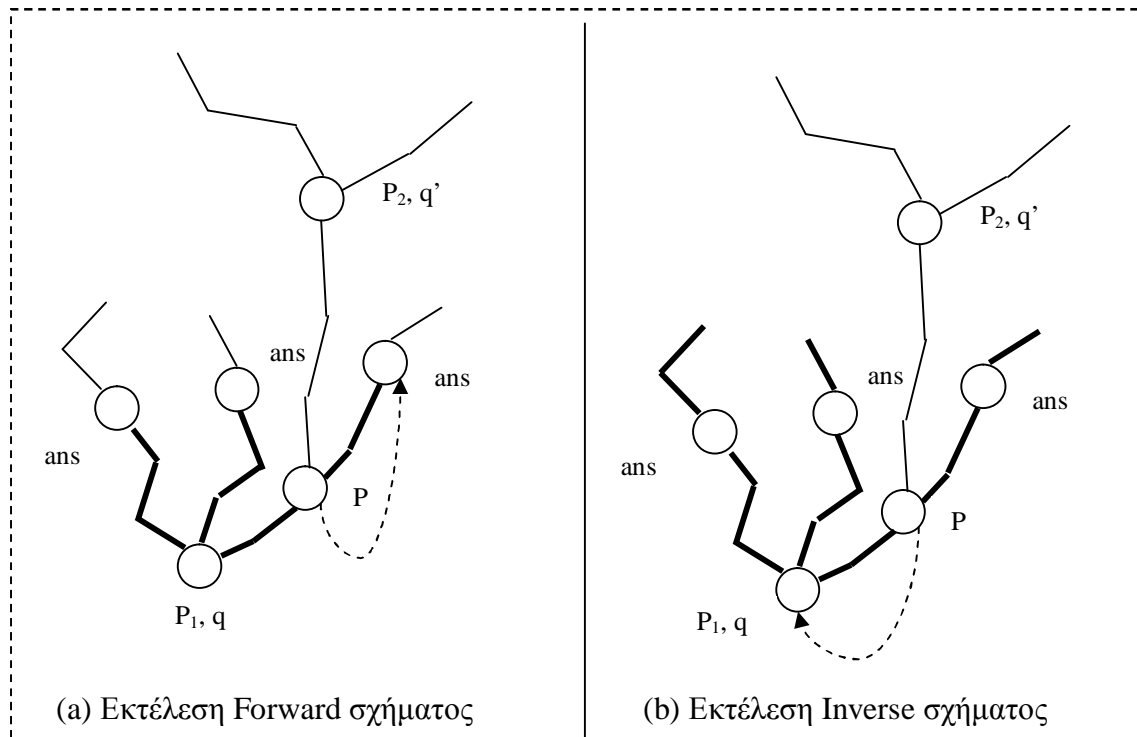
Σχήμα 2.4 Ο P_1 υποβάλλει την q μια χρονική στιγμή t_1 . Την χρονική στιγμή t_2 > t_1 ο P_2 υποβάλλει την q' παρόμοια της q . Σε αυτό το περιβάλλον θεωρούμε ότι οι ερωτήσεις είναι διάσημες. Στα αριστερά απεικονίζεται η εκτέλεση των ερωτημάτων στο Forward ή ηχανισμό ενώ στα δεξιά στο Inverse. Με ans συμβολίζονται οι κόμβοι απάντησης ενώ με έντονη γραμμή απεικονίζονται οι ονοπάτια στα οποία οι κόμβοι εισάγουν στην cache ένα ερώτημα
