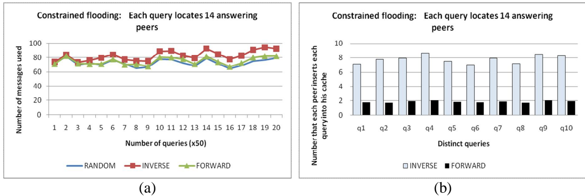
Σχήμα 3.9 Το Q.S είναι το ίδιο που χρησιμοποιήθηκε στο πείραμα 3.3.4. Το \lambda έγεθος της αναζήτησης που πετυχαίνουν οι τεχνικές για κάθε μια ερώτηση είναι συγκρίσιμο με το πείραμα 3.3.4
