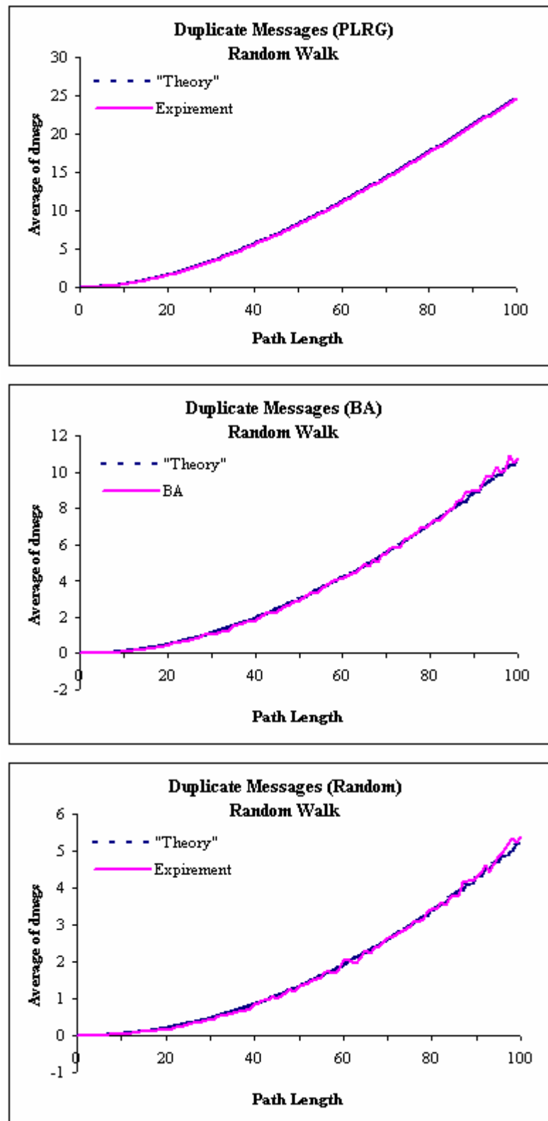
Σχήμα 6.13: Σύγκριση αναλυτικών και πειραματικών αποτελεσμάτων ως προς τα διπλά μηνύματα που παράγονται σε διάφορες τοπολογίες.
