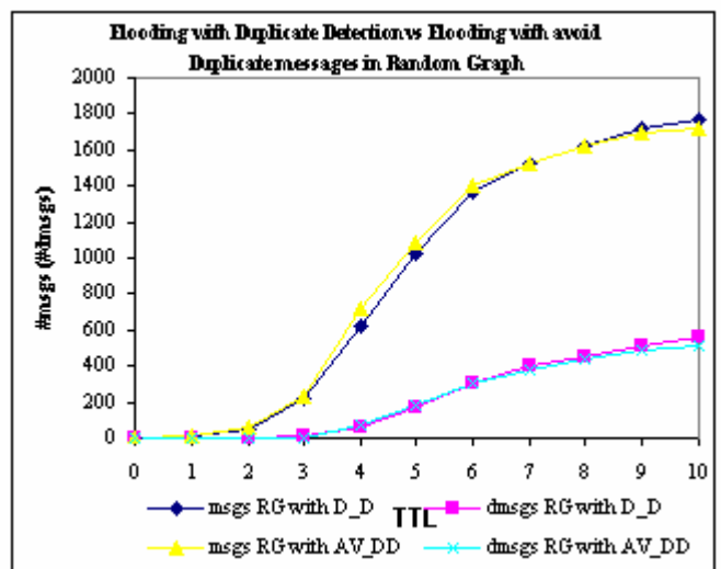
Σχήμα 6.15: Σύγκριση της πλημμύρας με DD και της πλημμύρας με DD και αποφυγή διπλών μηνυμάτων (AV) [32] στις τοπολογίες PLRG, BA, Random σε ασύγχρονο δίκτυο.
