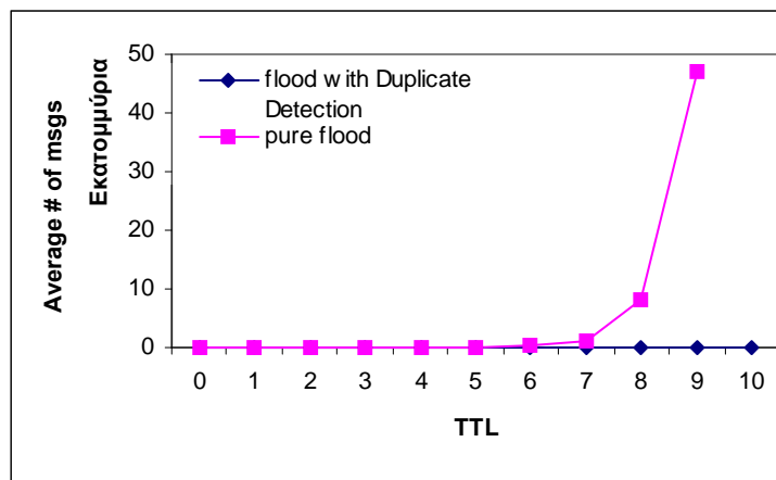
Σχήμα 4.3: Αναζήτηση με πλημμύρα σε δίκτυο με τοπολογία Barabasi, 1000 κόμβων. Ο συνολικός αριθμός μηνυμάτων με πλημμυρά (pure flooding) μειώνεται έως και 100% με εφαρμογή μηχανισμού duplicate detection.
