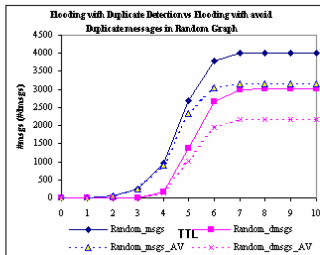
Σχήμα 6.14: Σύγκριση της πλημμύρας με DD και της πλημμύρας με DD και αποφυγή διπλών μηνυμάτων (AV) [32] στις τοπολογίες PLRG, BA, Random σε σύγχρονο δίκτυο.
