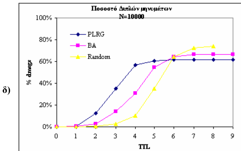
Σχήμα 6.5: Μέσο πλήθος παραγόμενων συνολικών μηνυμάτων και μέσο πλήθος συνολικών διπλών μηνυμάτων σε δίκτυα των 1000 κόμβων (α, β) αντίστοιχα και σε δίκτυα των 10000 κόμβων (γ, δ) αντίστοιχα.
