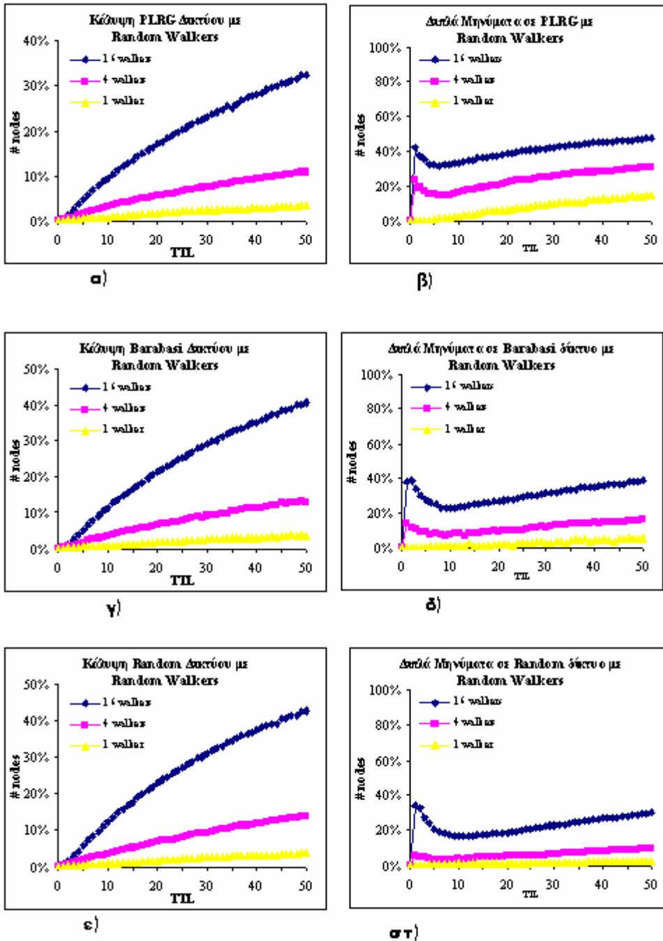
Σχήμα 6.11: Ποσοστό κάλυψης δικτύων με 1, 4 και 16 random walks και ποσοστό διπλών μηνυμάτων σε δίκτυο 1000 κόμβων σε σχέση με το χρόνο TTL και για τις τρεις διαφορετικές τοπολογίες (PLRG, BA, Random Graph).
