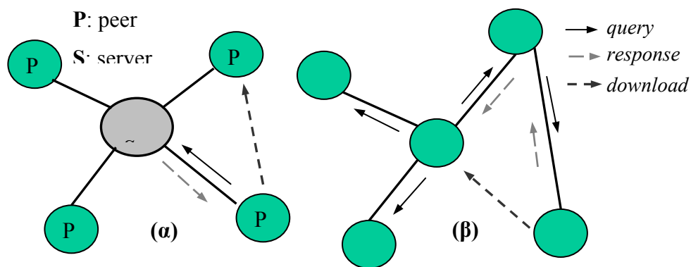
Σχήμα 4.1: Διαδικασία εκτέλεσης της αναζήτησης σε κεντροποιημένο σύστημα, όπως (α) στο Napster και (β) σε αδόμητο σύστημα όπως η Gnutella.
