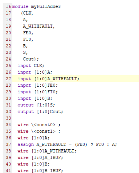
Σχήμα Γ.10 - Το netlist αρχείο, έτσι όπως φαίνεται στο source files
