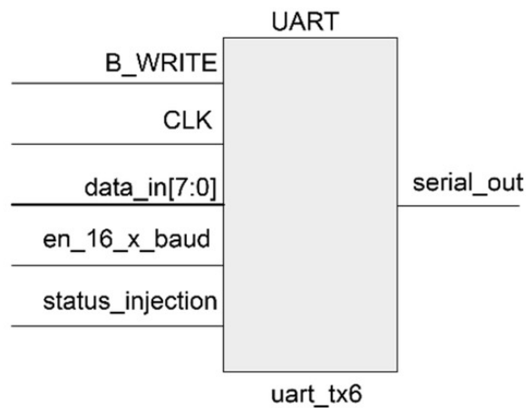
Σχήμα B.1 - Το pinout της μονάδας UART του FPGA
