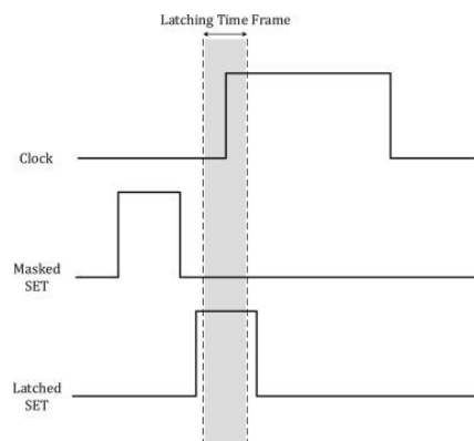
Σχήμα 2.2 - Παρουσία σφάλματος σε ένα κύκλωμα. Μη ανιχνεύσιμο λόγω του timing masking effect [11]
