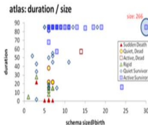
Σχήμα 3-6 - The Γ pattern -- από το [VaZS16] με άδεια των συγγραφέων – σελ 29
