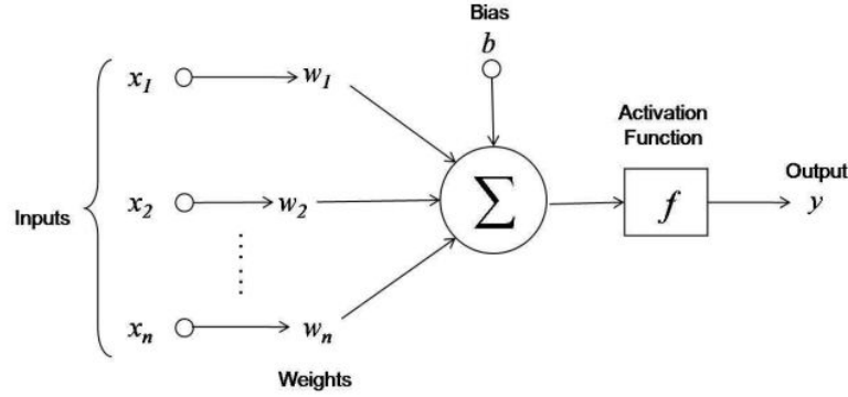
Σχήμα 2.2: Τεχνητός Νευρώνας
