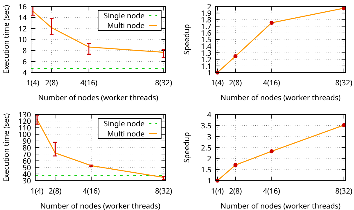
Σχήμα 6.3: Επάνω: Διάγραμμα χρόνου εκτέλεσης του προγράμματος Matmul σε διαφορετικά πλήθη κόμβων (αριστερά) και επιτάχυνσης (δεξιά) για πίνακες μεγέθους 1024x1024. Κάτω: Διάγραμμα χρόνου εκτέλεσης (αριστερά) και επιτάχυνσης (δεξιά) για πίνακες μεγέθους 2048x2048.
