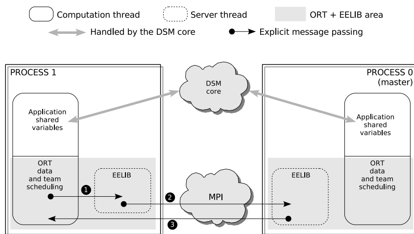
Σχήμα 3.3: Η οργάνωση της υπάρχουσας υποδομής για clusters στον OMPI. Οι μεταβλητές του προγράμματος του χρήστη γίνονται κοινόχρηστες με τη βοήθεια των βιβλιοθηκών sDSM, όπως φαίνεται στο επάνω μισό. Αντίθετα, οι μεταβλητές της υλοποίησης του ORT γίνονται κοινόχρηστες μέσω ρητών κλήσεων στο MPI, όπως φαίνεται στο σκιασμένο μέρος. Το Σχήμα αυτό προέρχεται από το [15].
