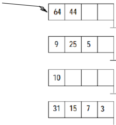
Εικόνα 1: Πίνακας γραμμικού κατακερματισμού
